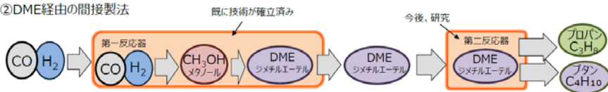
②DME経由の間接製法
