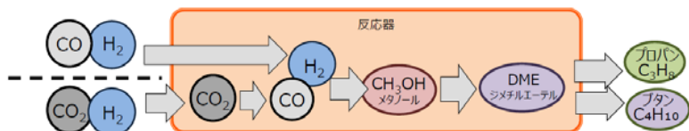
②DME経由の間接製法
